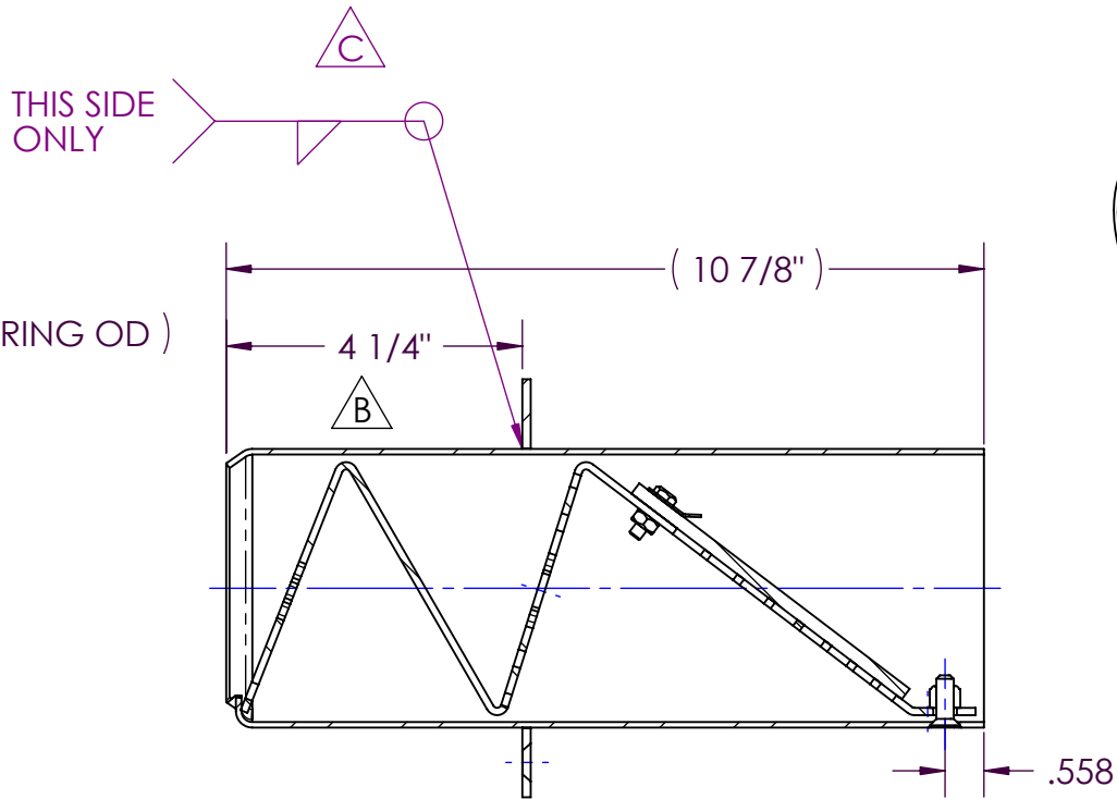
SECTION A-A
